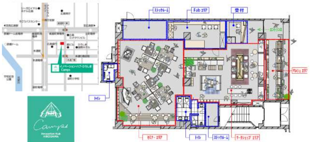
【平面図】
